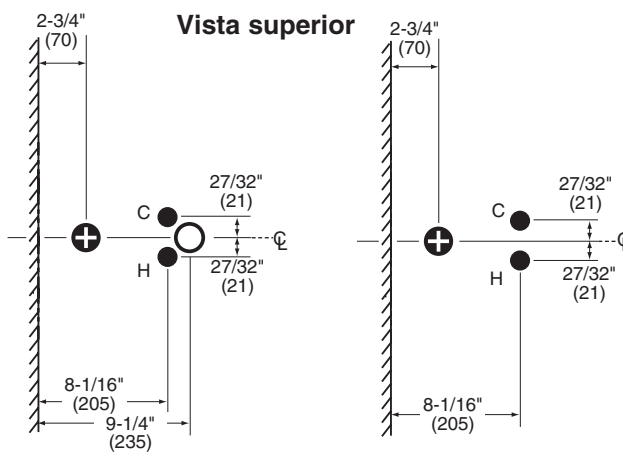
Tipo B Ventilación ascendente desde el centro (el sifón en P viene con la unidad).
